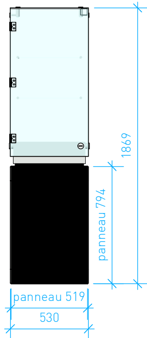
Vue face
