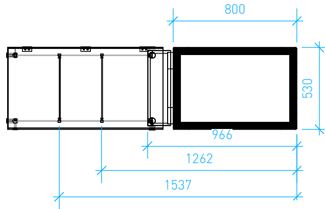
Vue gauche
